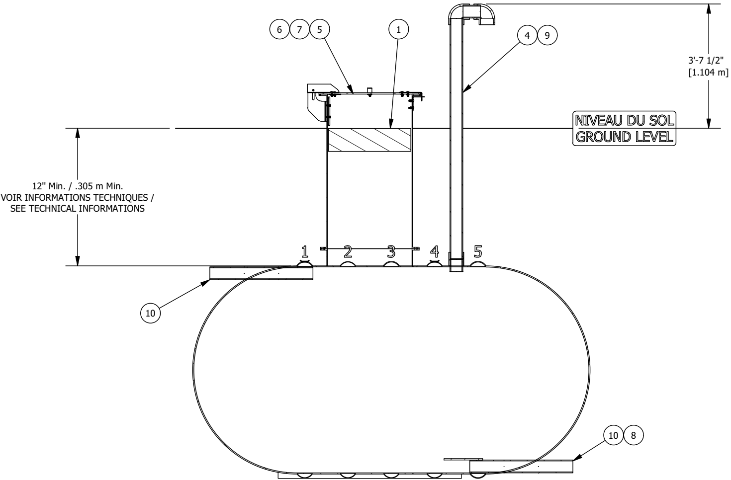
VUE D'ÉLEVATION COUPÉE CUT ELEVATION VIEW
