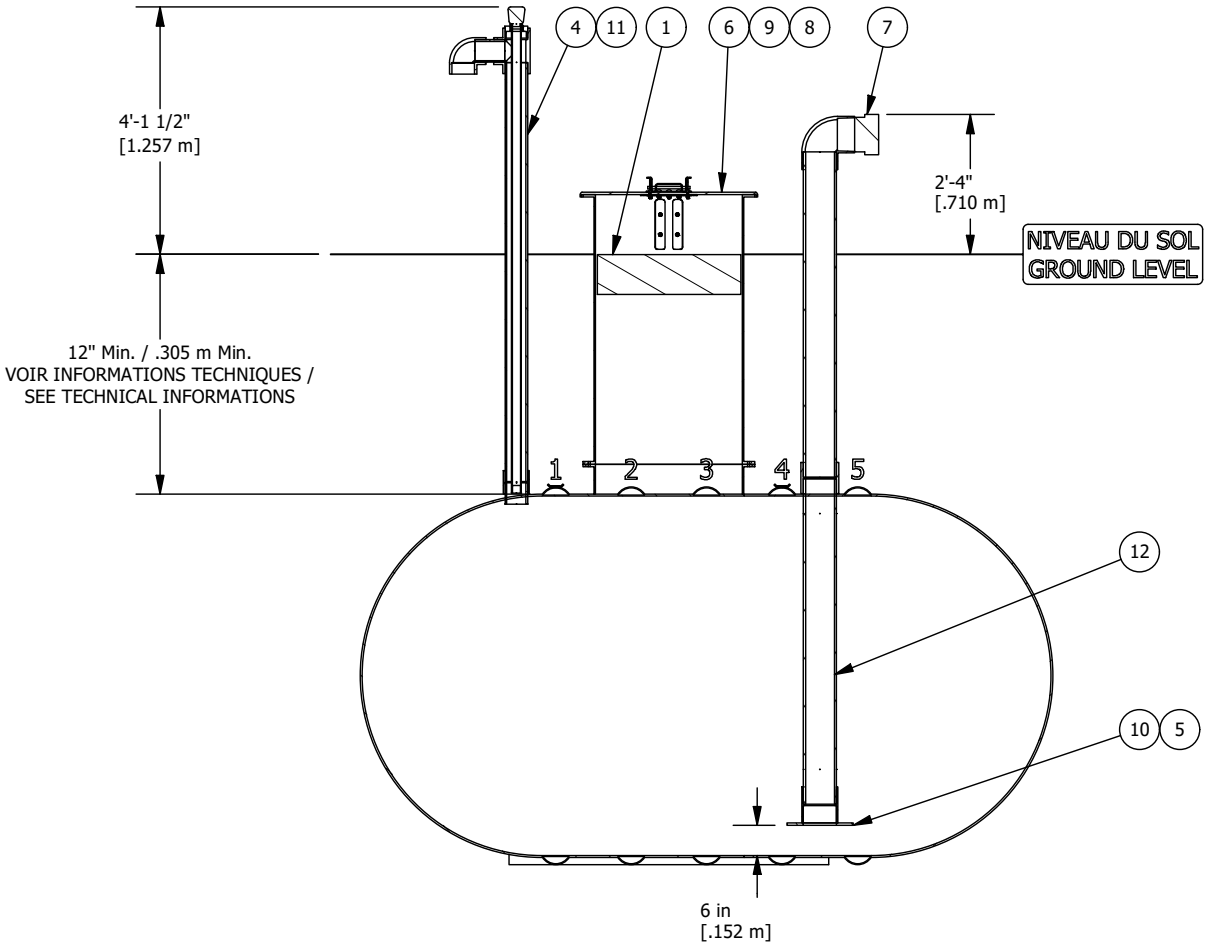
VUE D'ÉLEVATION COUPÉE CUT ELEVATION VIEW
