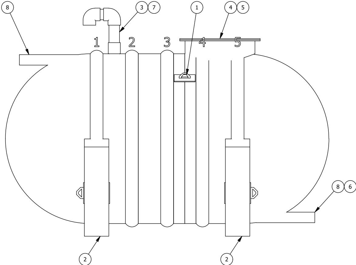
VUE D'ÉLÉVATION ELEVATION VIEW
