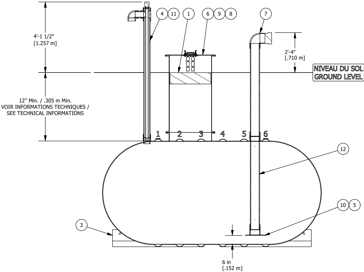
VUE D'ÉLEVATION COUPÉE CUT ELEVATION VIEW
