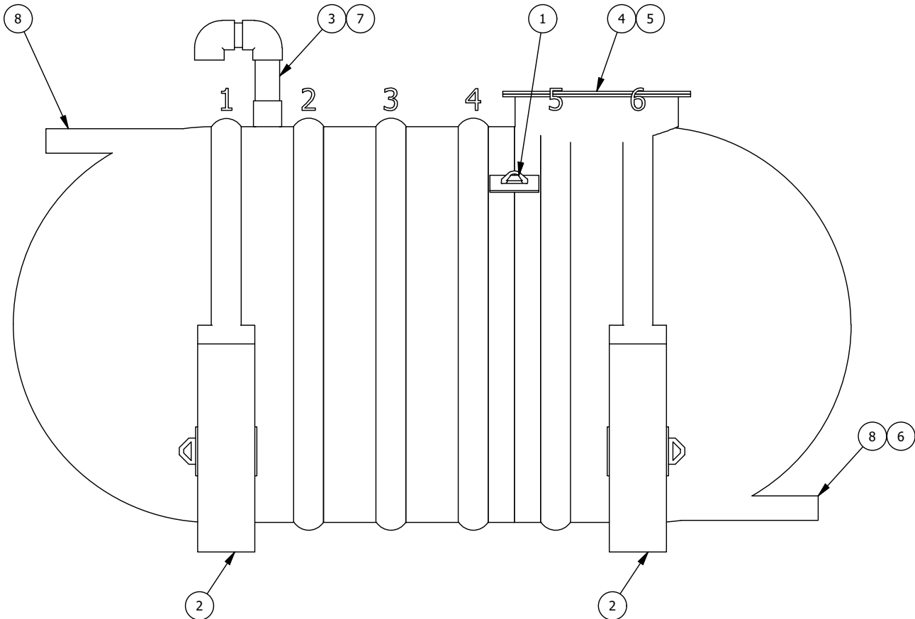
VUE D'ÉLEVATION ELEVATION VIEW
