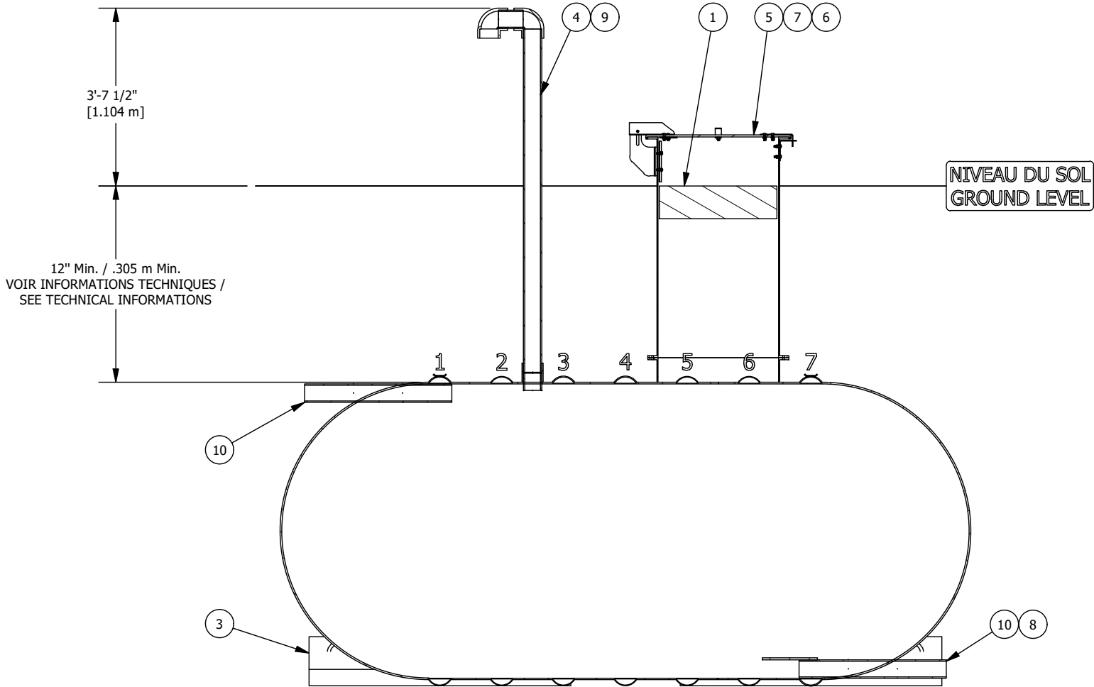
VUE D'ÉLEVATION COUPÉE CUT ELEVATION VIEW
