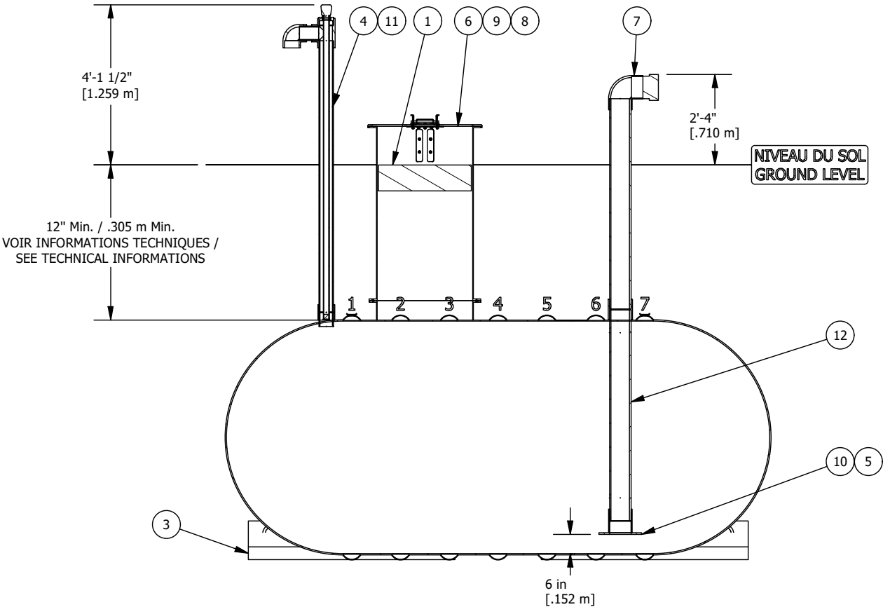
VUE D'ÉLEVATION COUPÉE CUT ELEVATION VIEW
