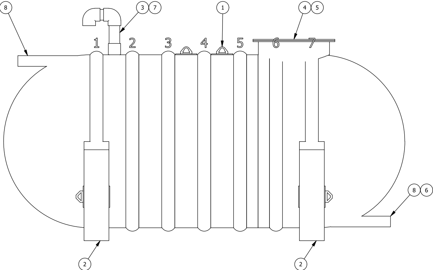
VUE D'ÉLÉVATION ELEVATION VIEW
