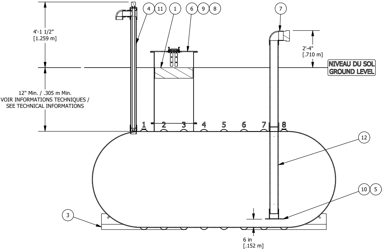
VUE D'ÉLEVATION COUPÉE CUT ELEVATION VIEW
