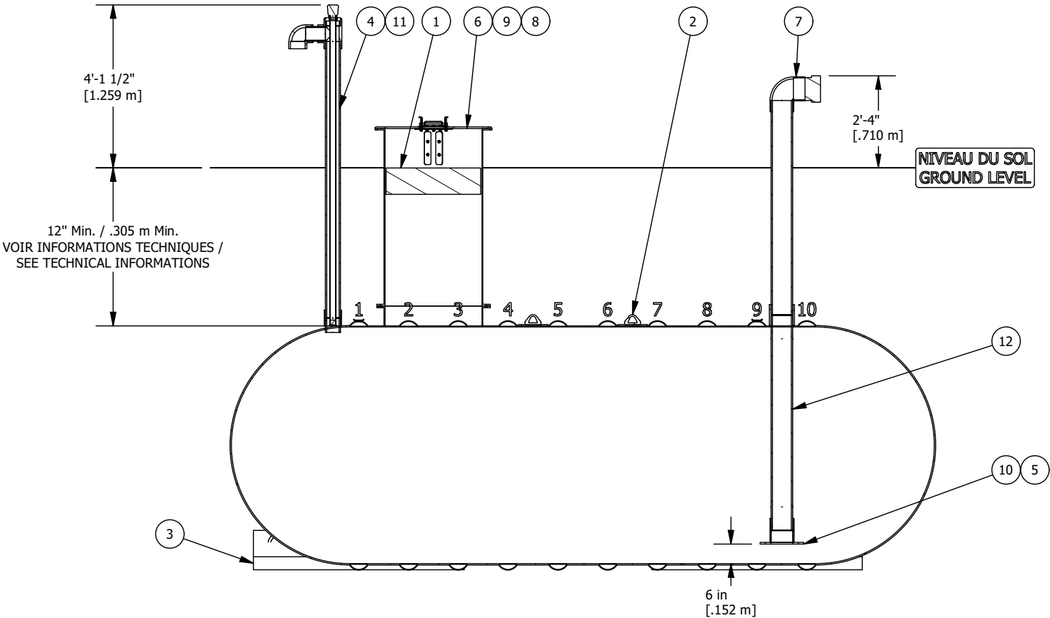
VUE D'ÉLEVATION COUPÉE CUT ELEVATION VIEW
