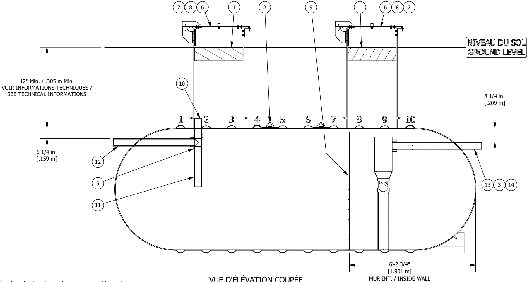
VUE D'ÉLEVATION COUPÉE CUT ELEVATION VIEW
