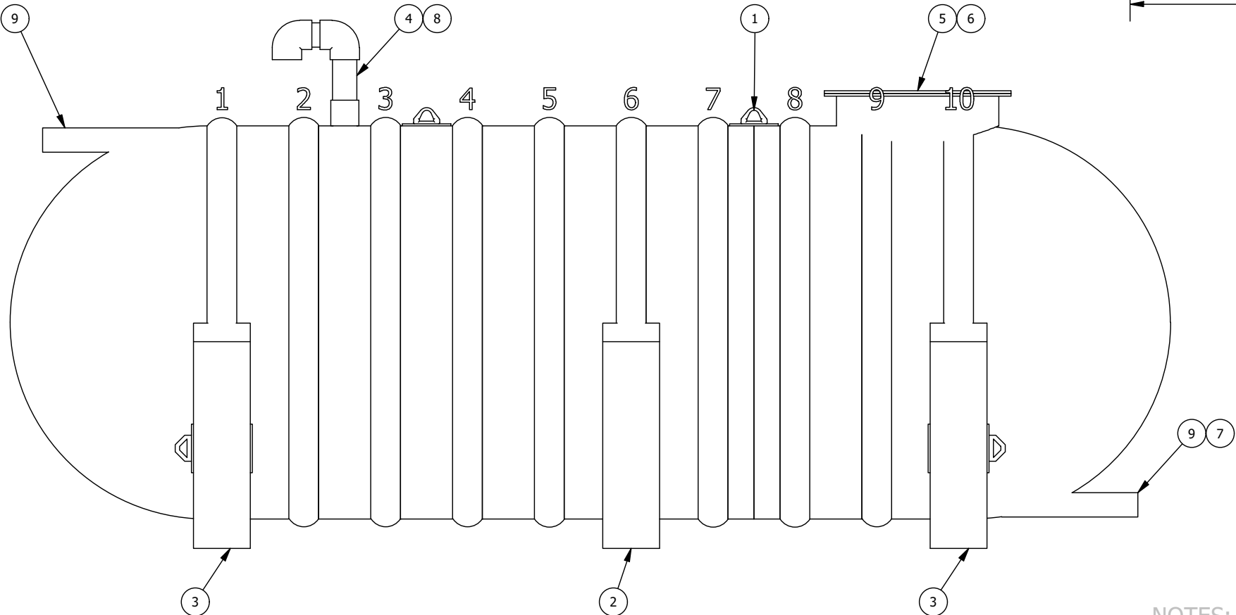
VUE D'ÉLÉVATION ELEVATION VIEW
