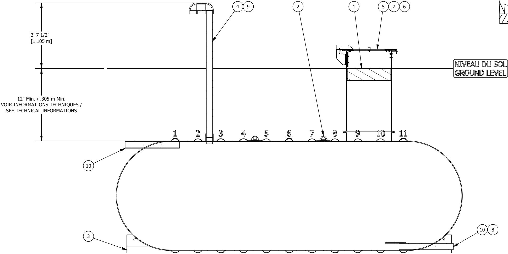
VUE D'ÉLEVATION COUPÉE CUT ELEVATION VIEW
