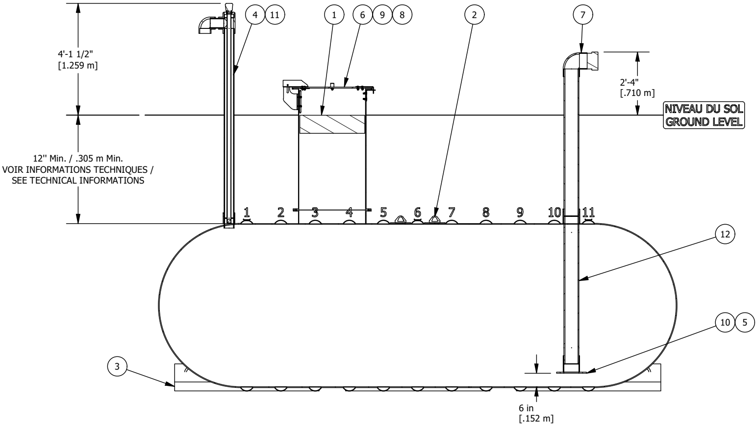
VUE D'ÉLEVATION COUPÉE CUT ELEVATION VIEW
