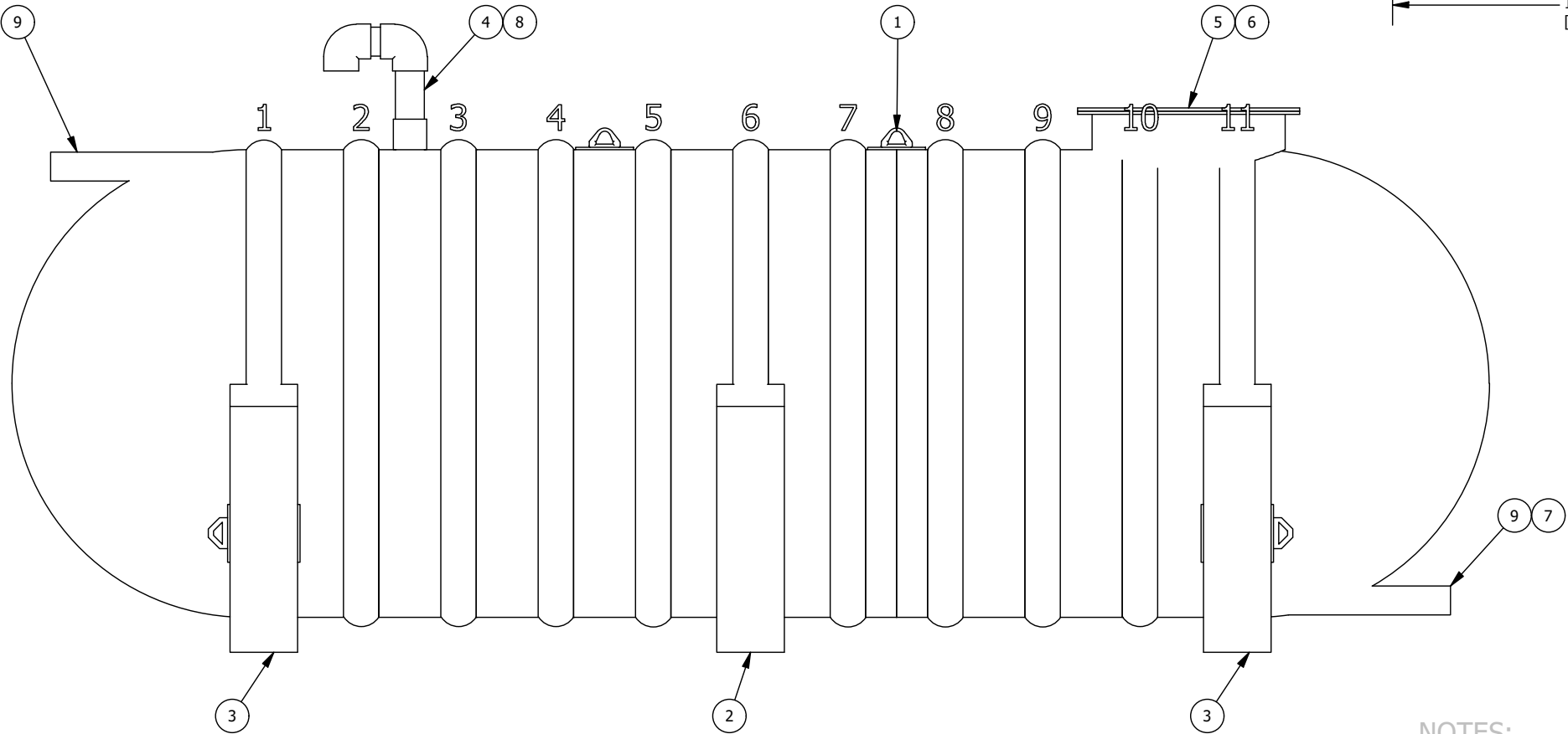
VUE D'ÉLÉVATION ELEVATION VIEW
