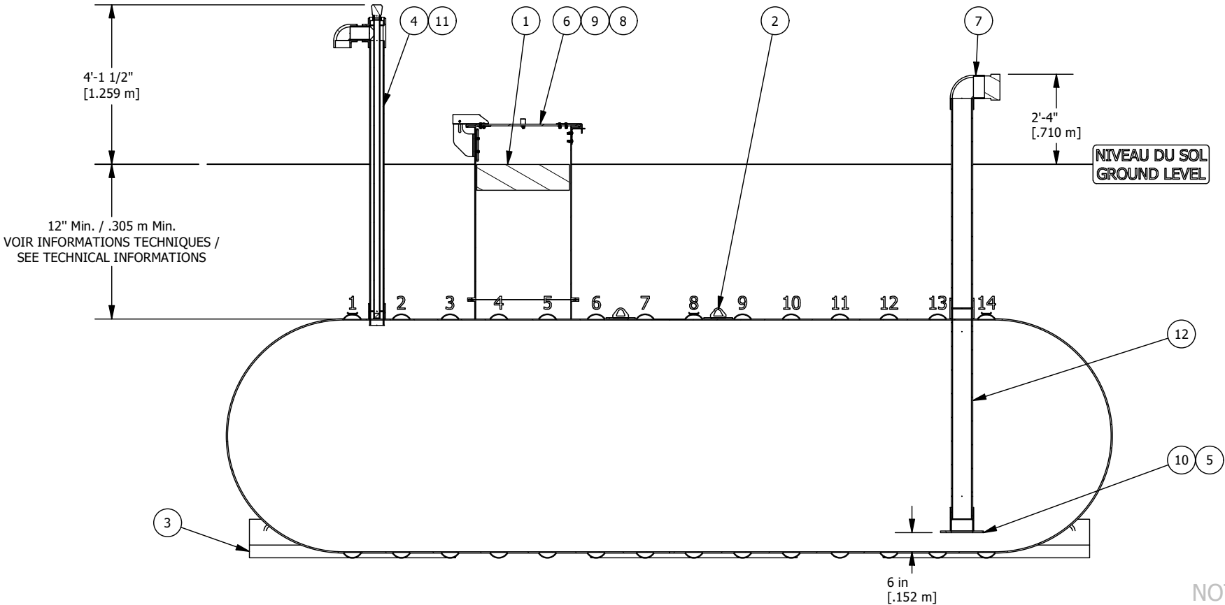
VUE D'ÉLÉVATION COUPÉE CUT ELEVATION VIEW
