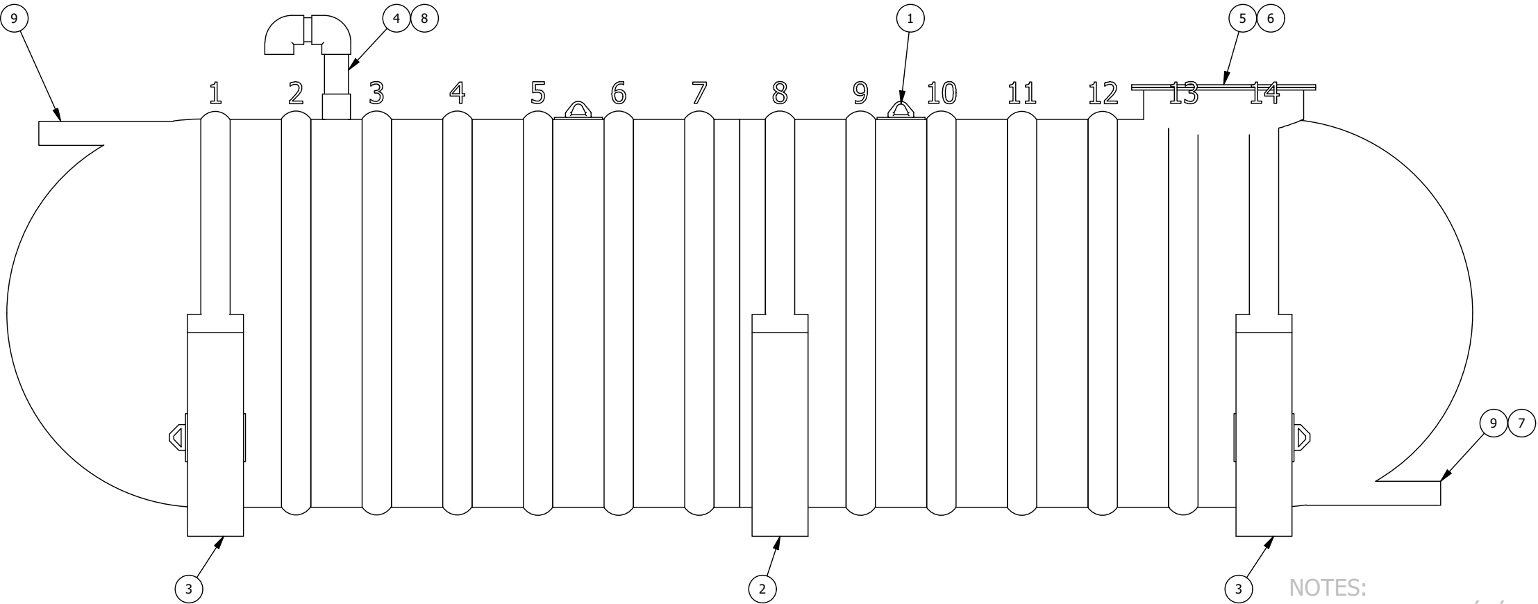
VUE D'ÉLÉVATION ELEVATION VIEW
