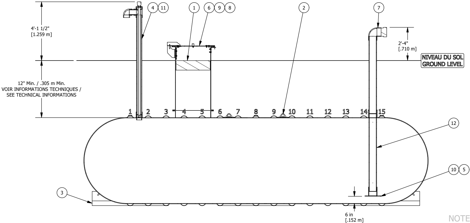
VUE D'ÉLÉVATION COUPÉE CUT ELEVATION VIEW
