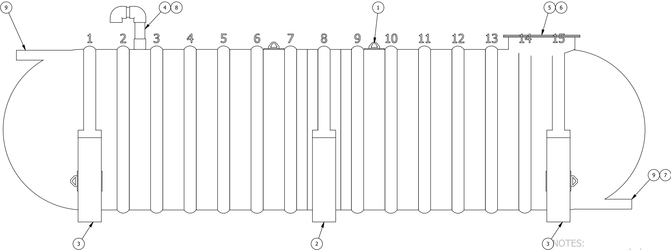
VUE D'ÉLÉVATION ELEVATION VIEW
