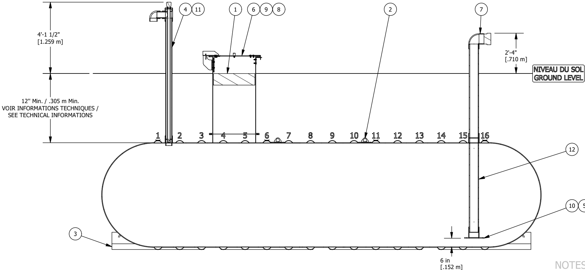
VUE D'ÉLEVATION COUPÉE CUT ELEVATION VIEW
