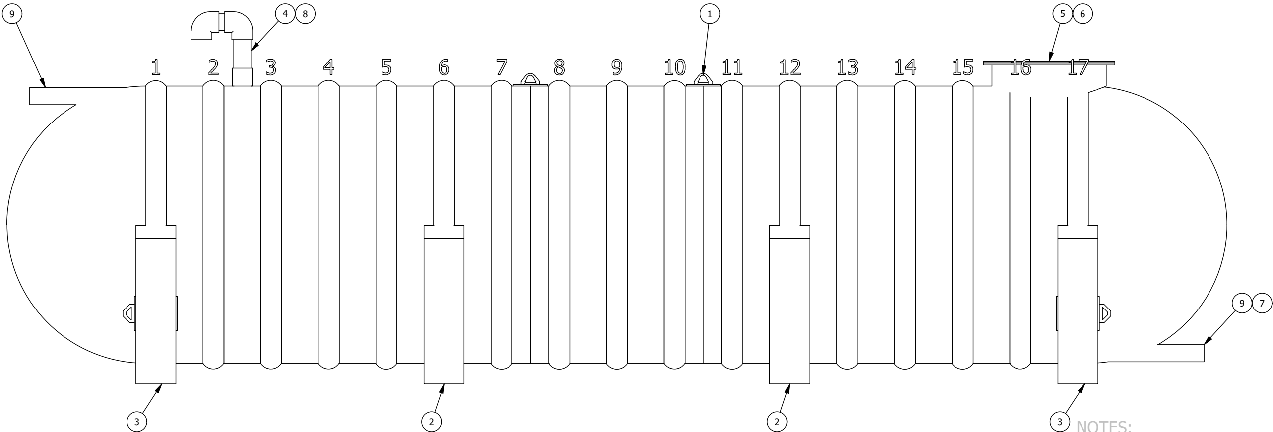
VUE D'ÉLÉVATION ELEVATION VIEW
