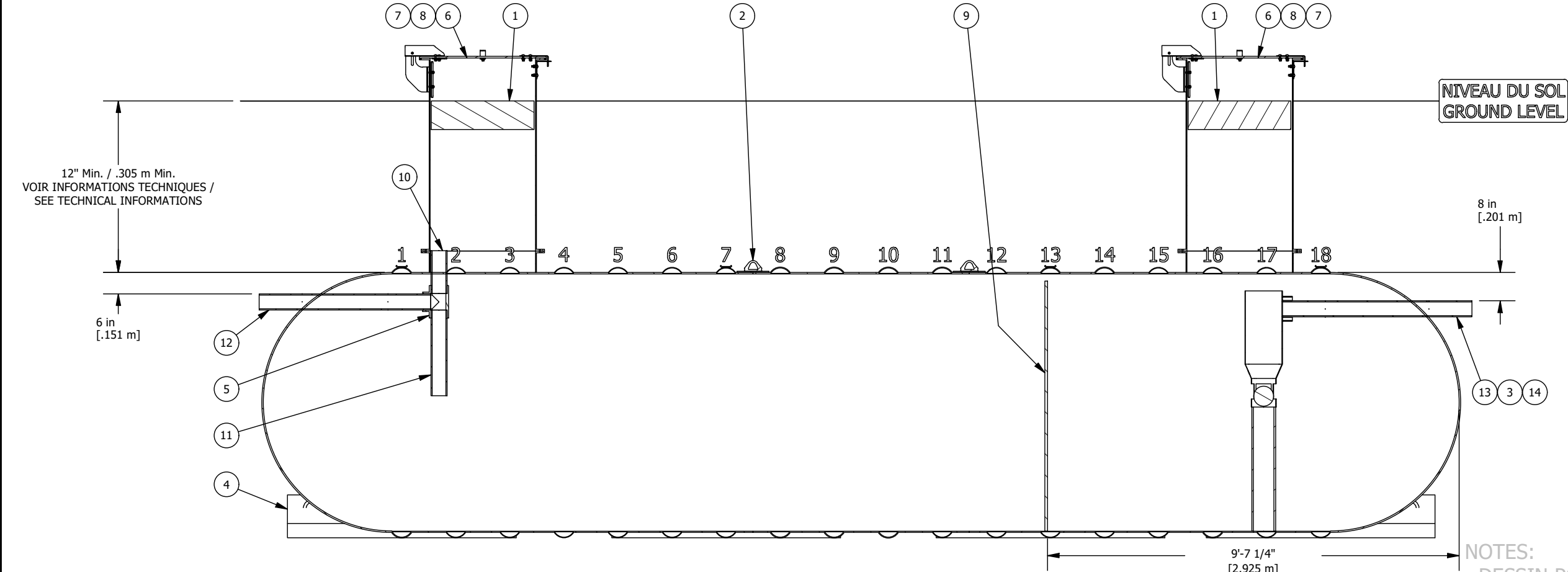
VUE D'ÉLEVATION COUPÉE CUT ELEVATION VIEW
