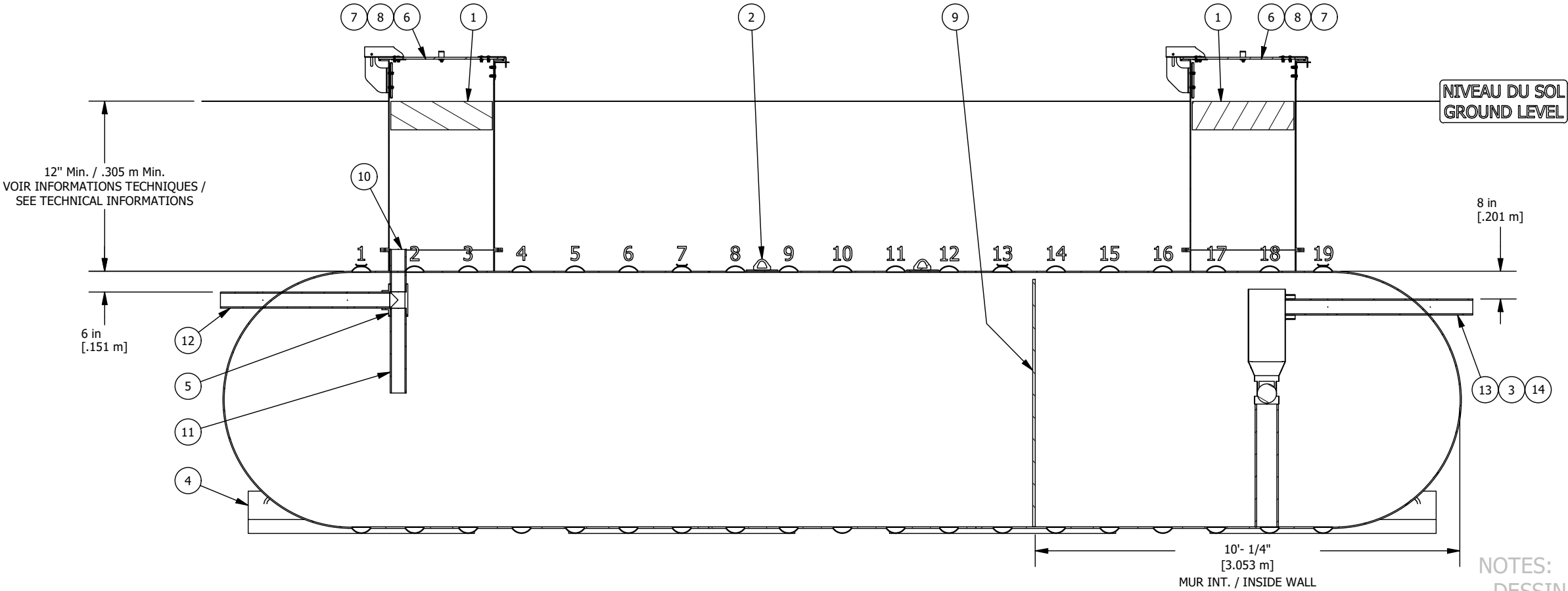
VUE D'ÉLEVATION COUPÉE CUT ELEVATION VIEW
