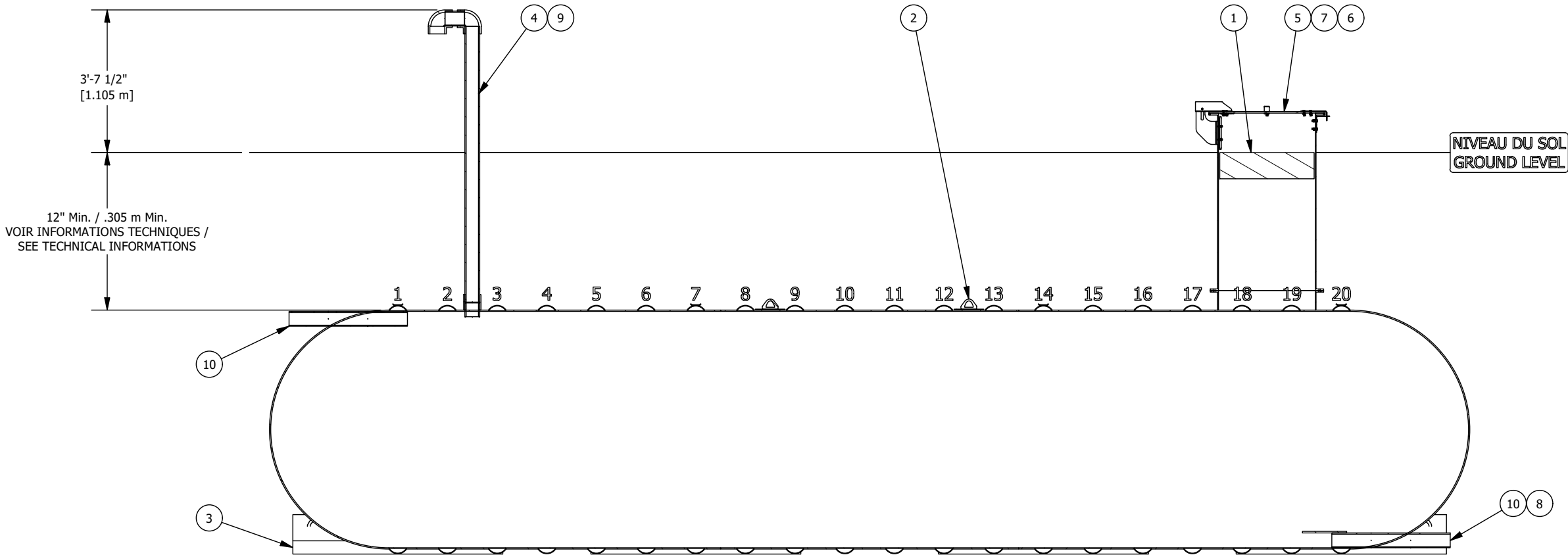
VUE D'ÉLEVATION COUPÉE CUT ELEVATION VIEW
