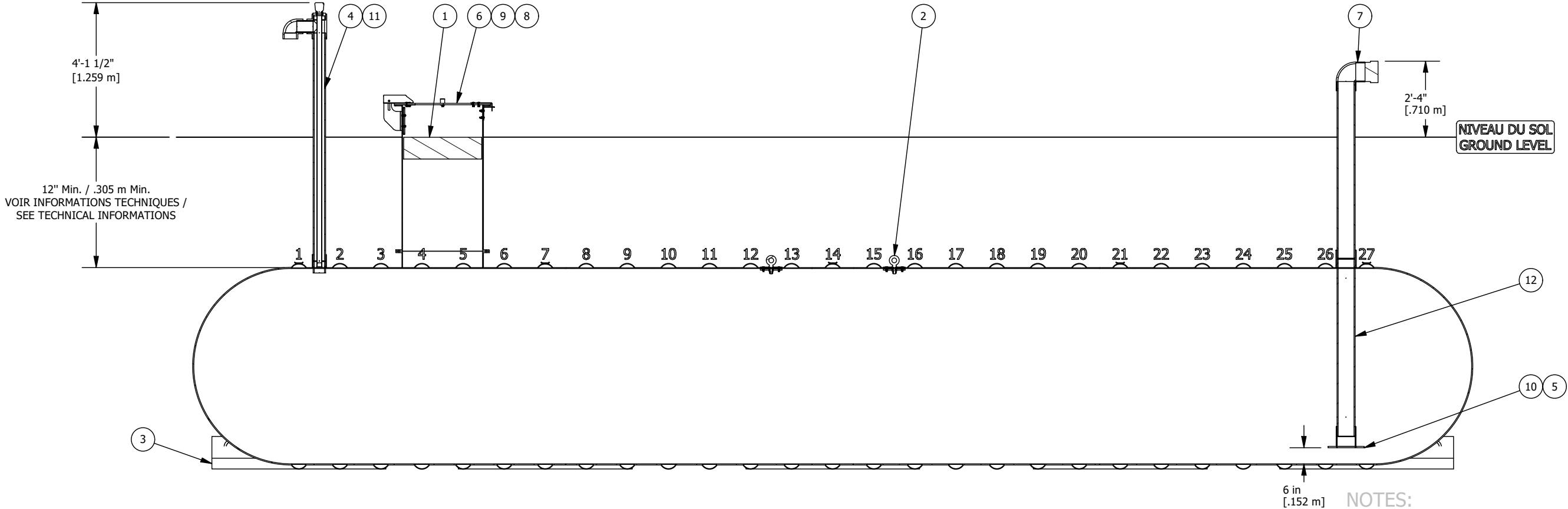
VUE D'ÉLEVATION COUPÉE CUT ELEVATION VIEW
