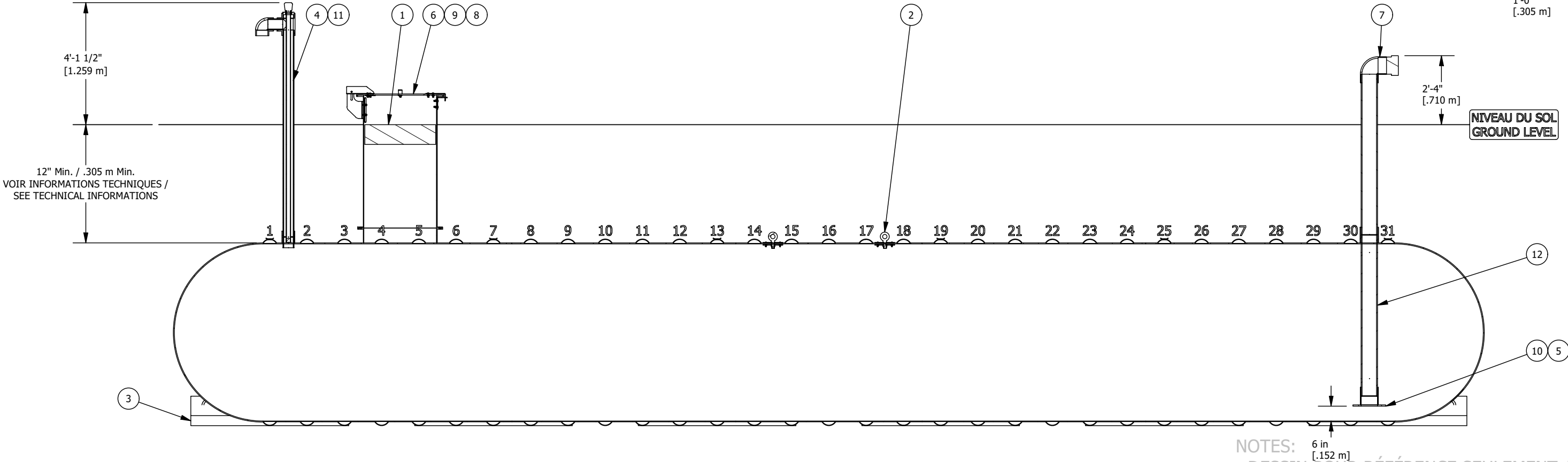
VUE D'ÉLEVATION COUPÉE CUT ELEVATION VIEW
