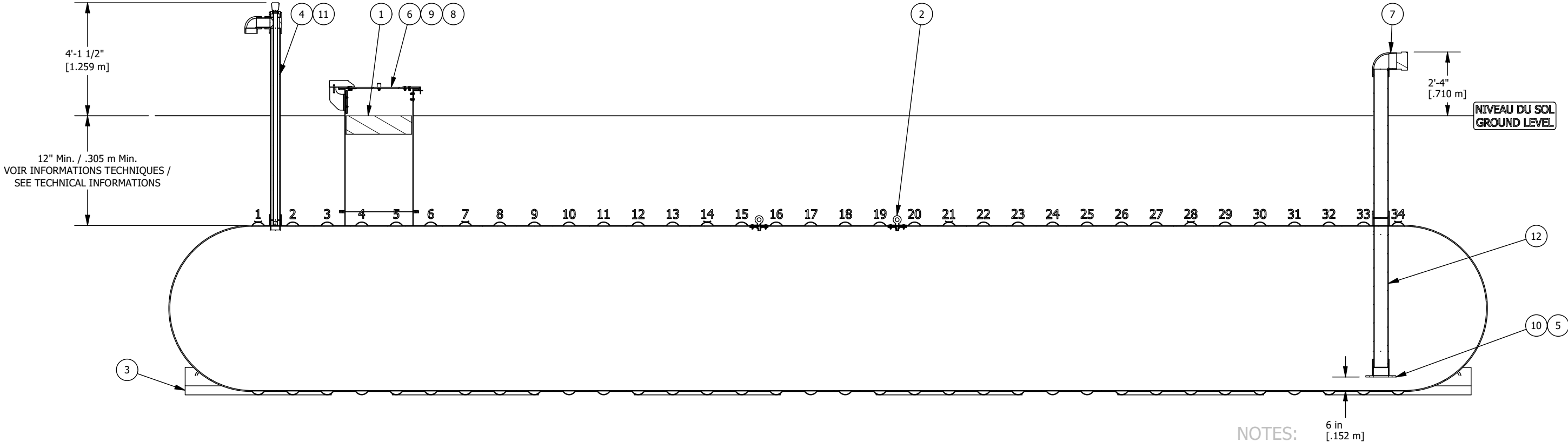
VUE D'ÉLEVATION COUPÉE CUT ELEVATION VIEW
