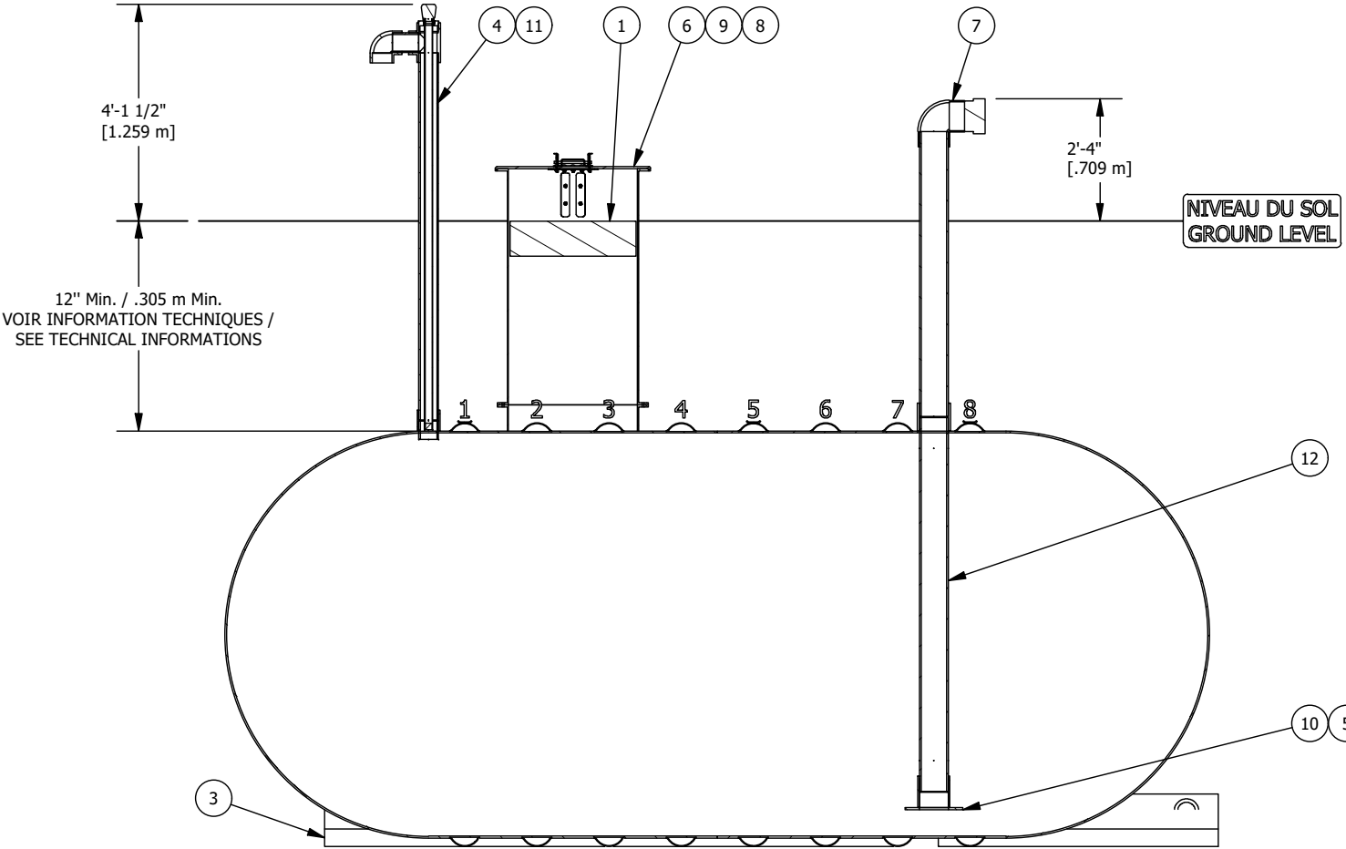
VUE D'ÉLEVATION COUPÉE CUT ELEVATION VIEW
