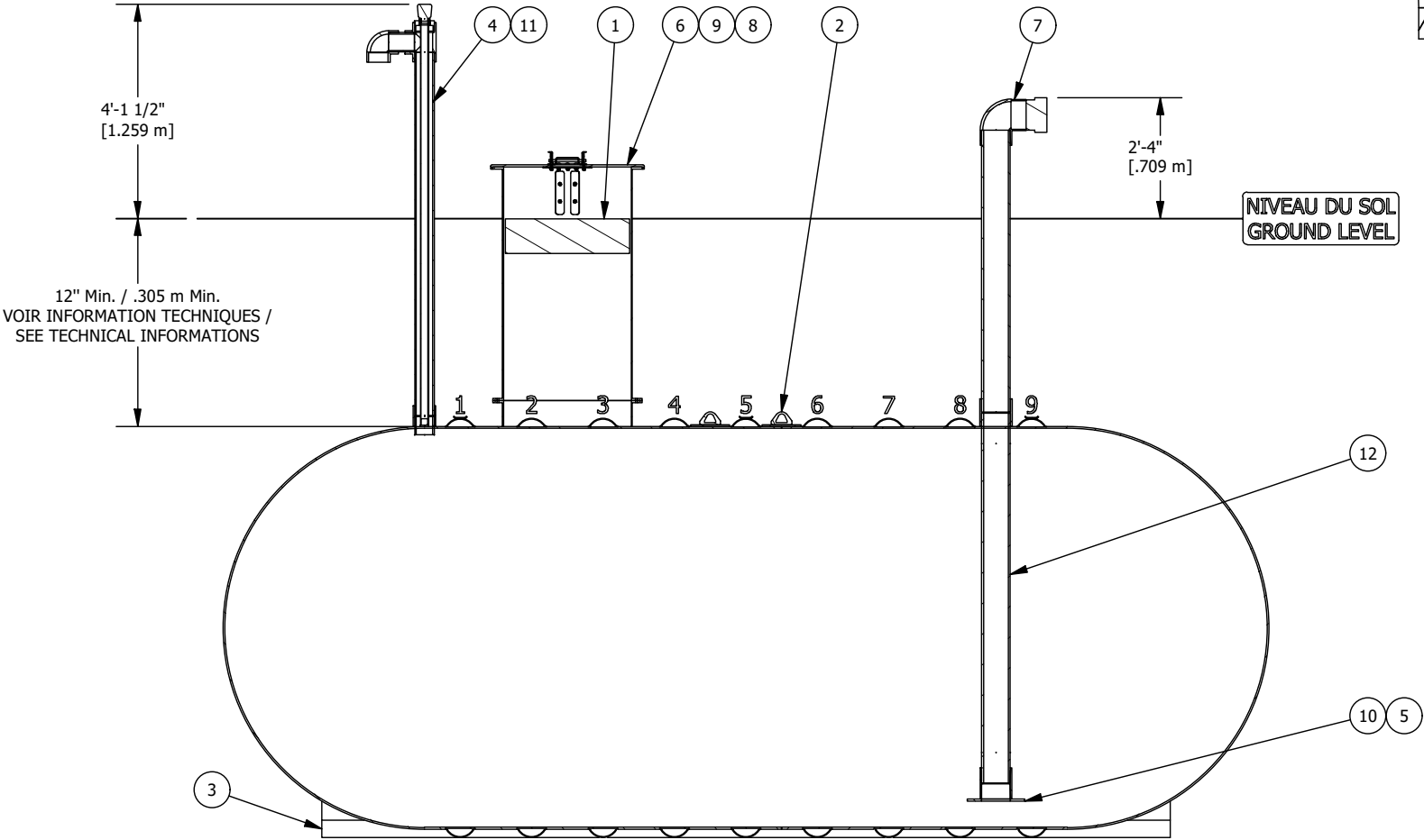
VUE D'ÉLEVATION COUPÉE CUT ELEVATION VIEW
