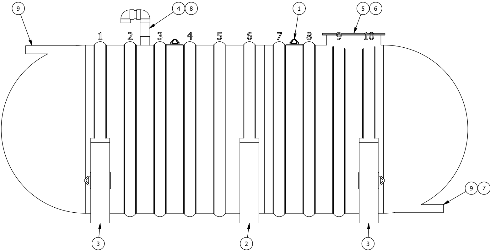
VUE D'ÉLÉVATION ELEVATION VIEW
