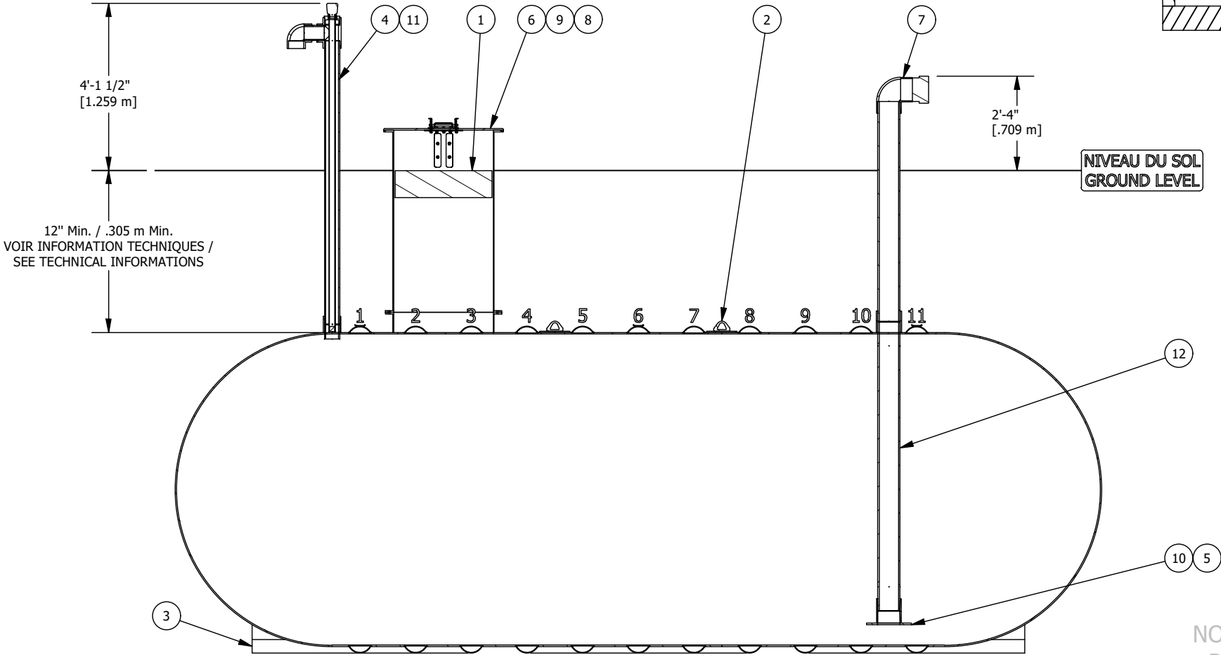
VUE D'ÉLÉVATION COUPÉE CUT ELEVATION VIEW
