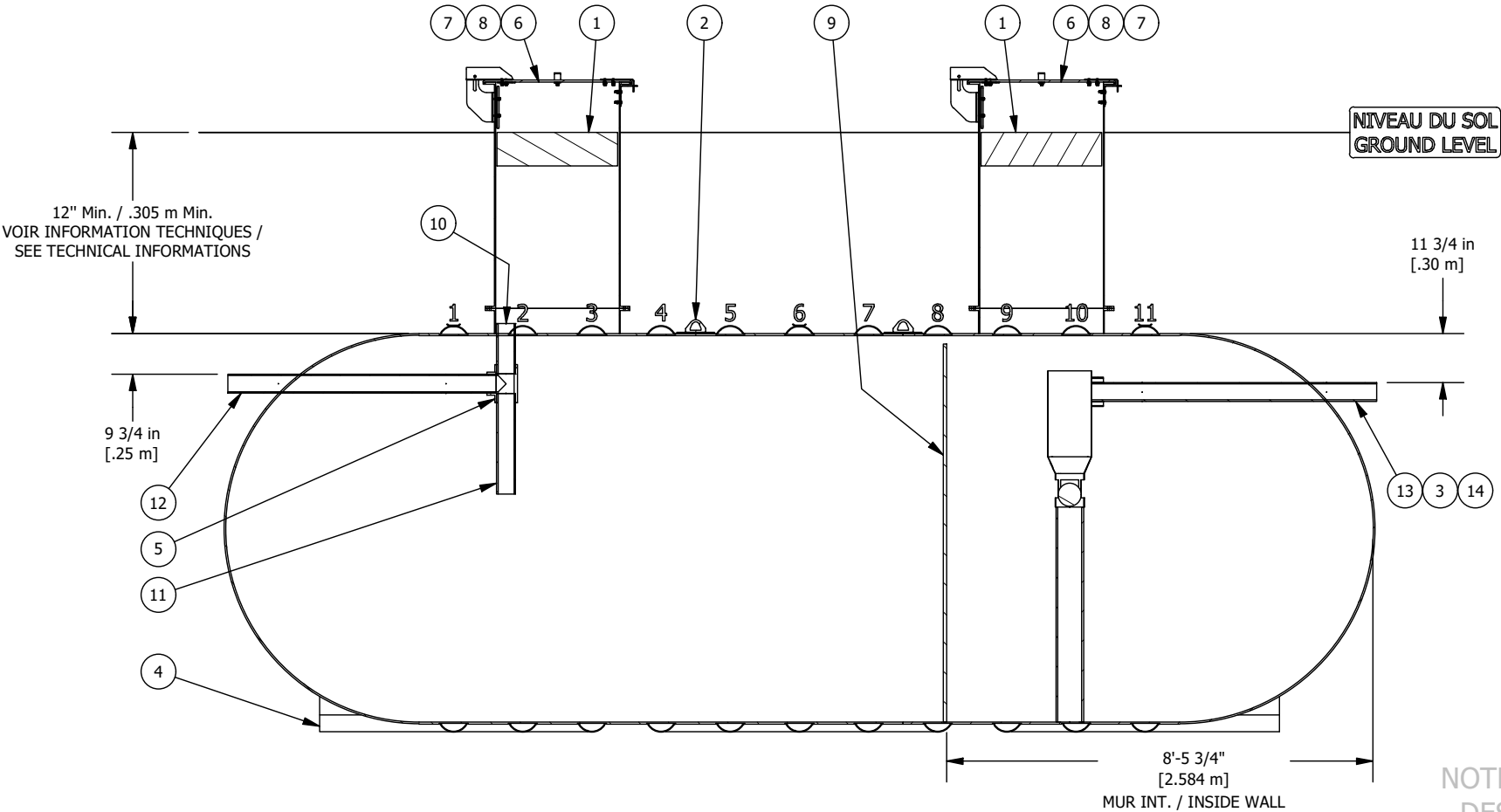
VUE D'ÉLEVATION COUPÉE CUT ELEVATION VIEW
