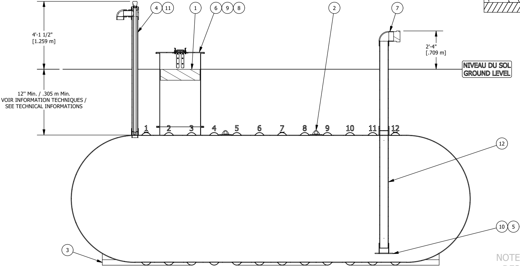
VUE D'ÉLEVATION COUPÉE CUT ELEVATION VIEW
