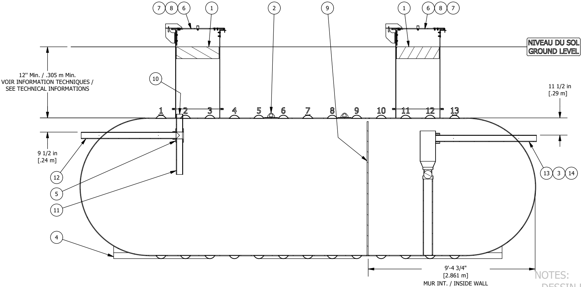
VUE D'ÉLEVATION COUPÉE CUT ELEVATION VIEW
