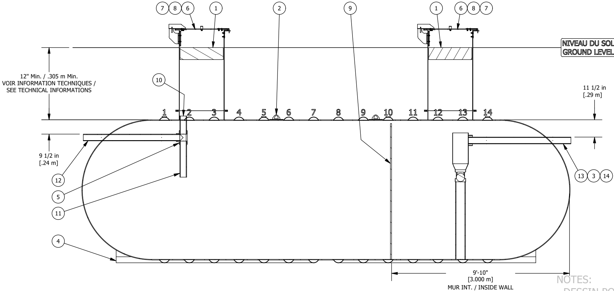
VUE D'ÉLEVATION COUPÉE CUT ELEVATION VIEW
