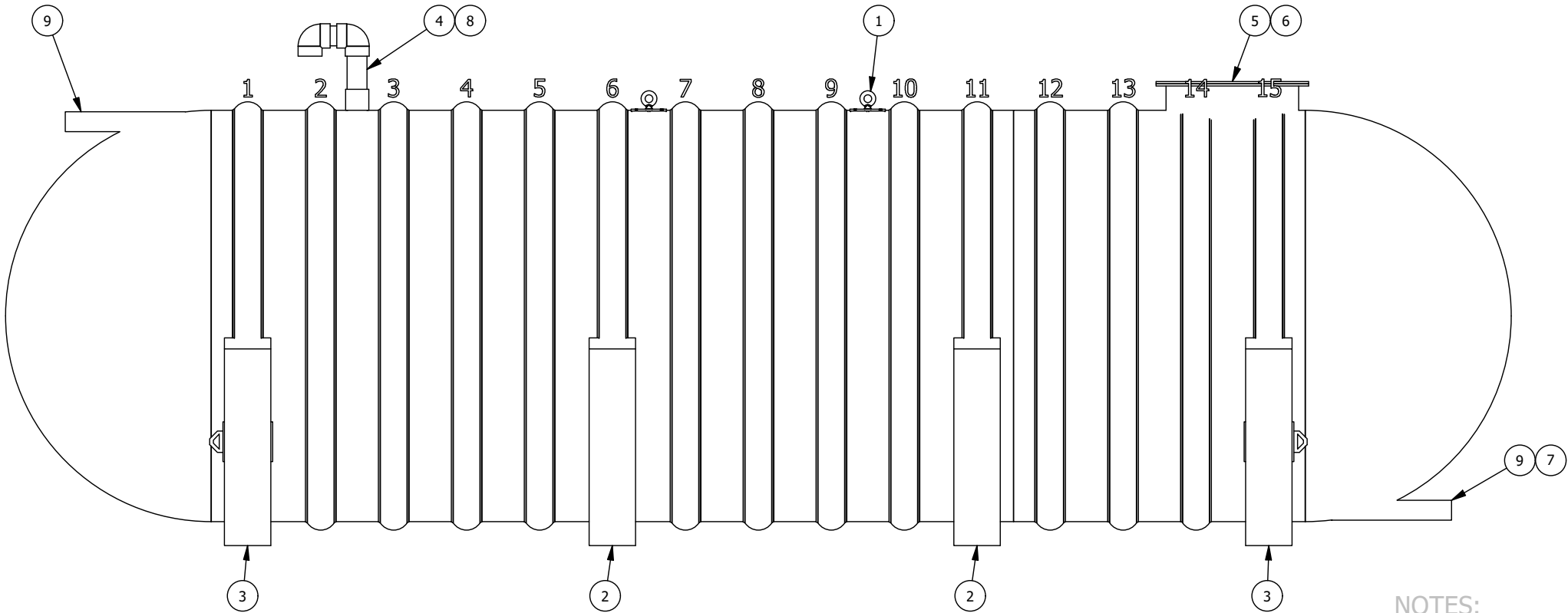
VUE D'ÉLÉVATION ELEVATION VIEW
