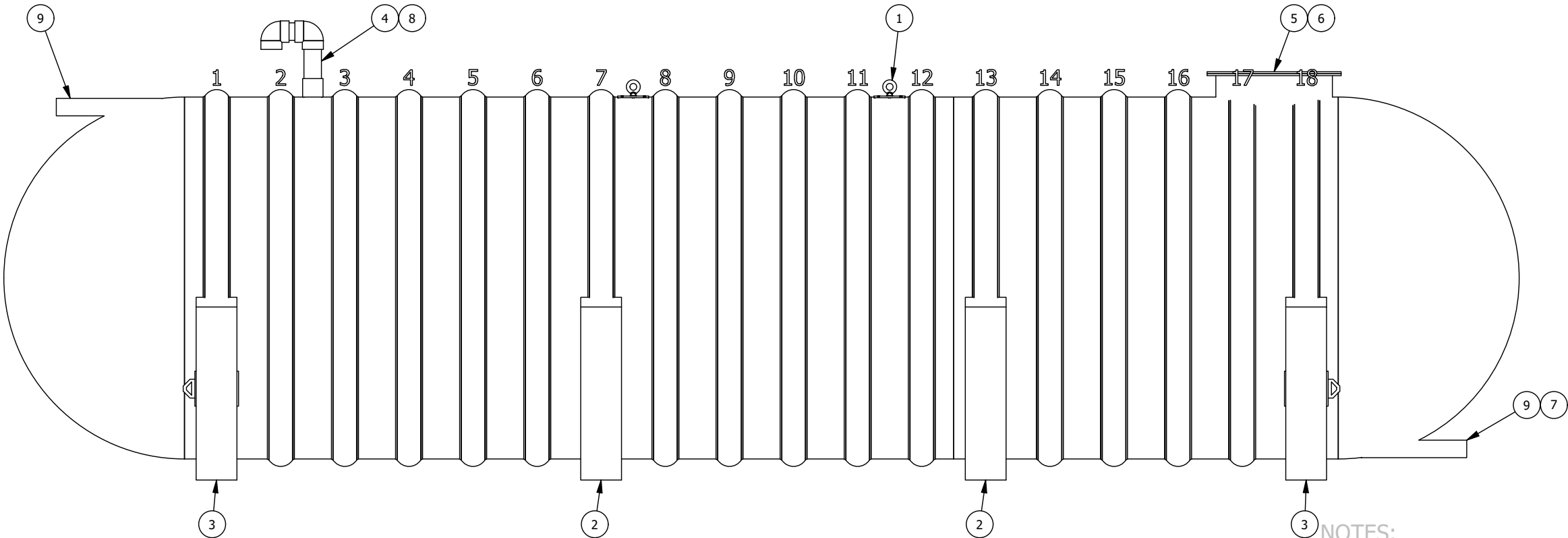
VUE D'ÉLÉVATION ELEVATION VIEW
