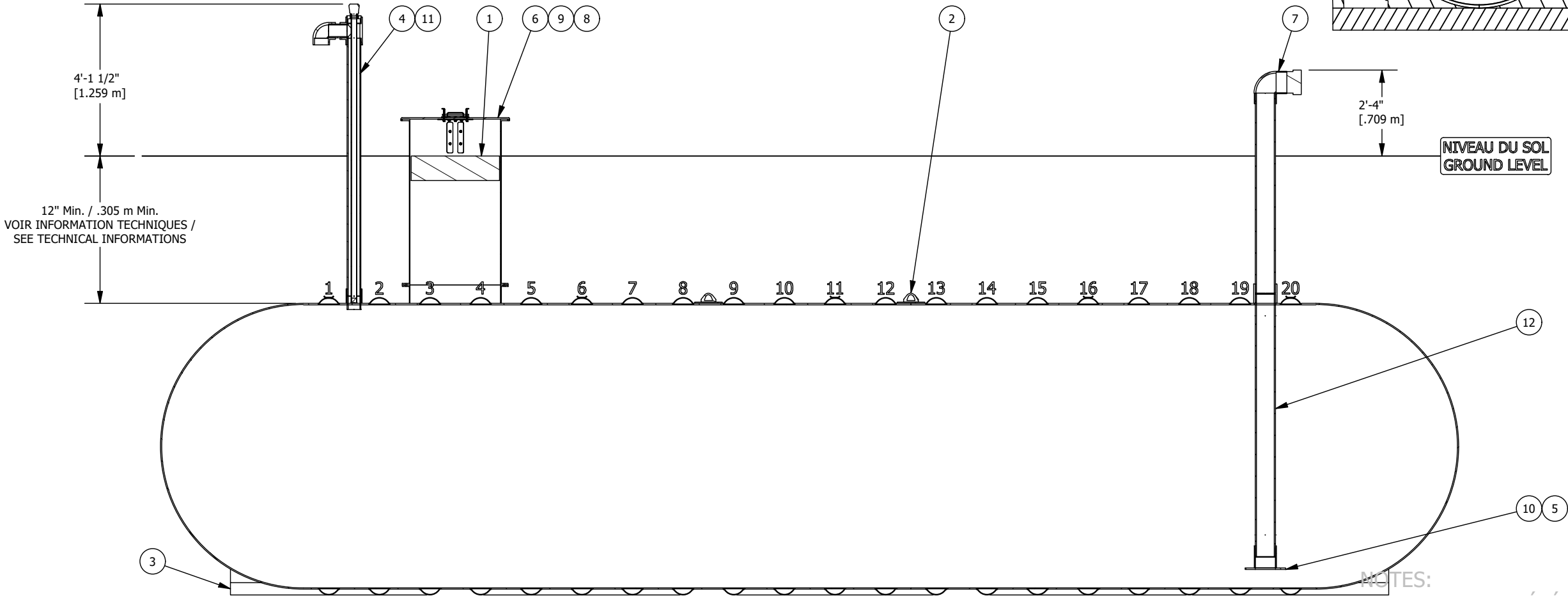
VUE D'ÉLEVATION COUPÉE CUT ELEVATION VIEW
