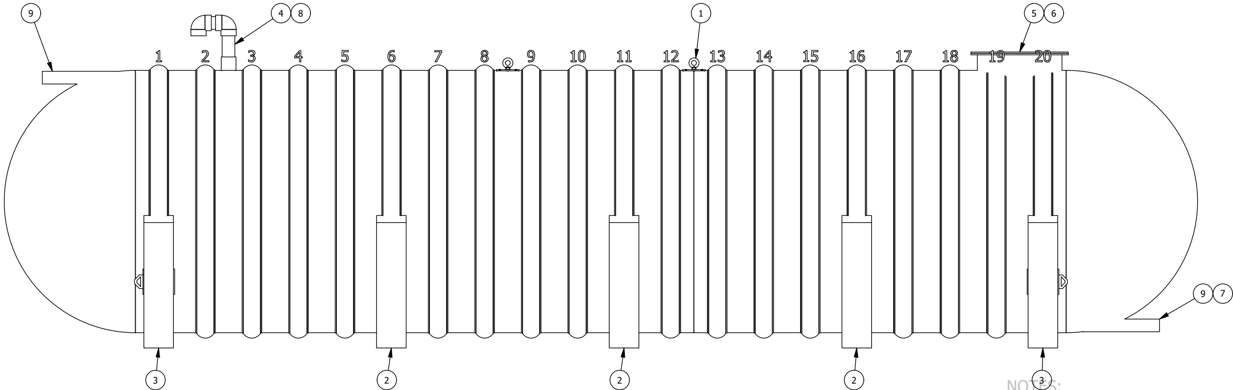
VUE D'ÉLEVATION ELEVATION VIEW
