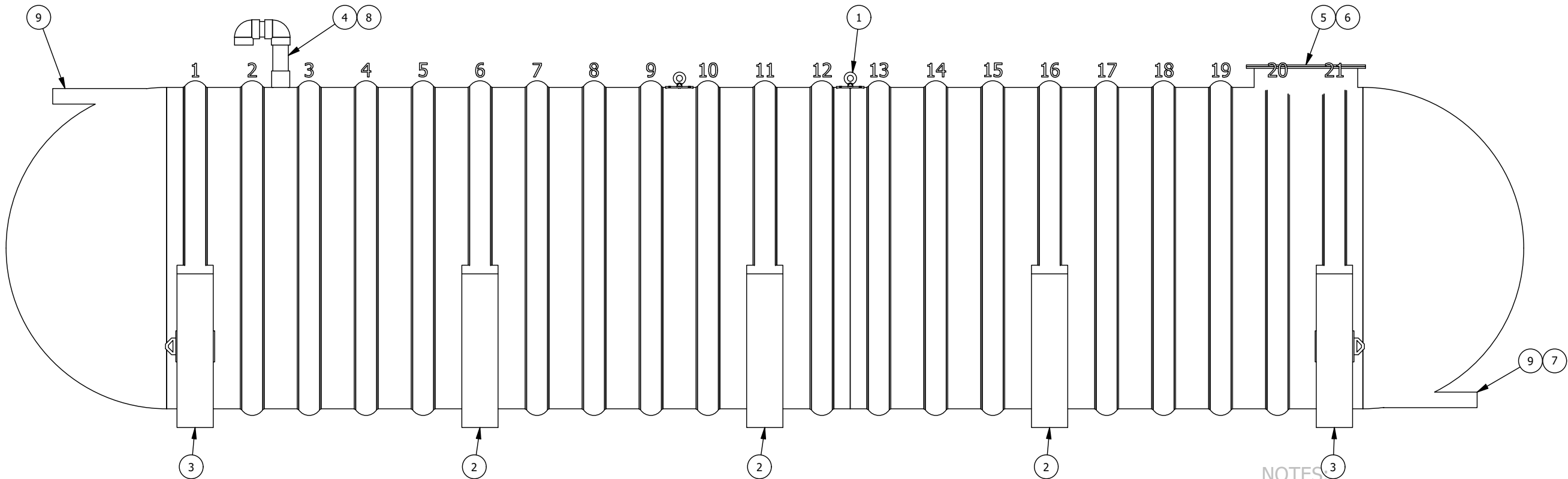
VUE D'ÉLÉVATION ELEVATION VIEW
