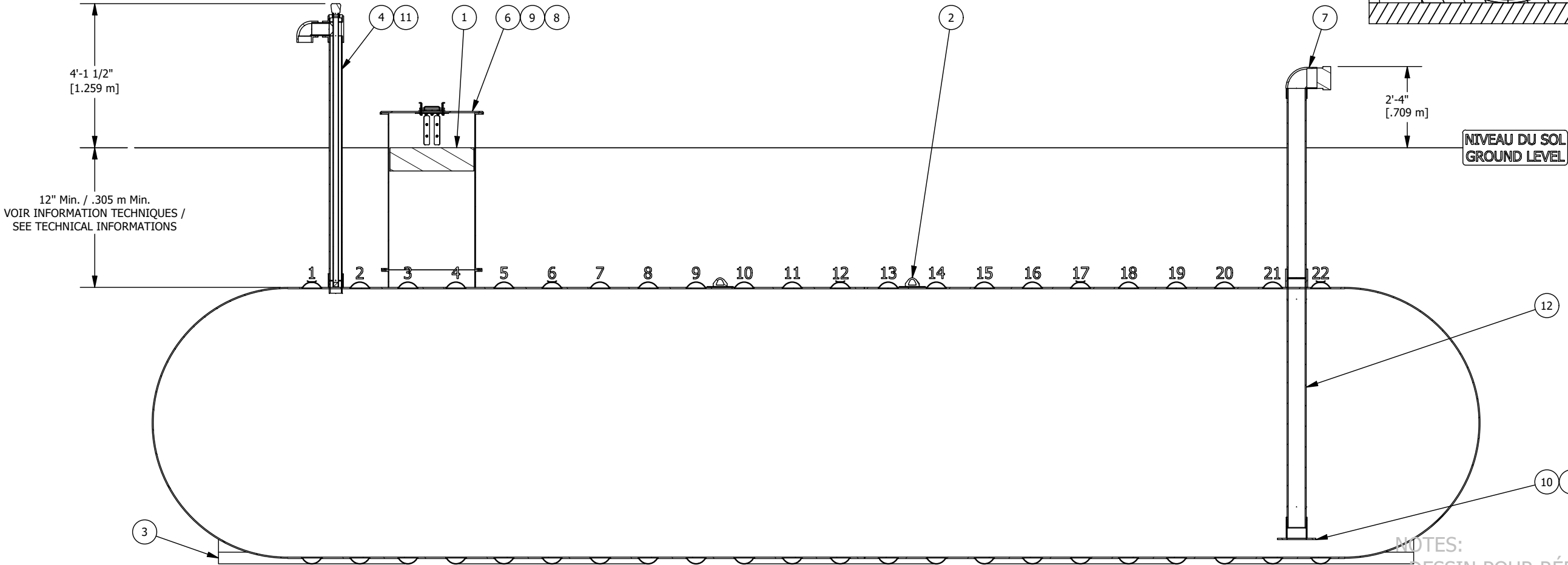
VUE D'ÉLEVATION COUPÉE CUT ELEVATION VIEW
