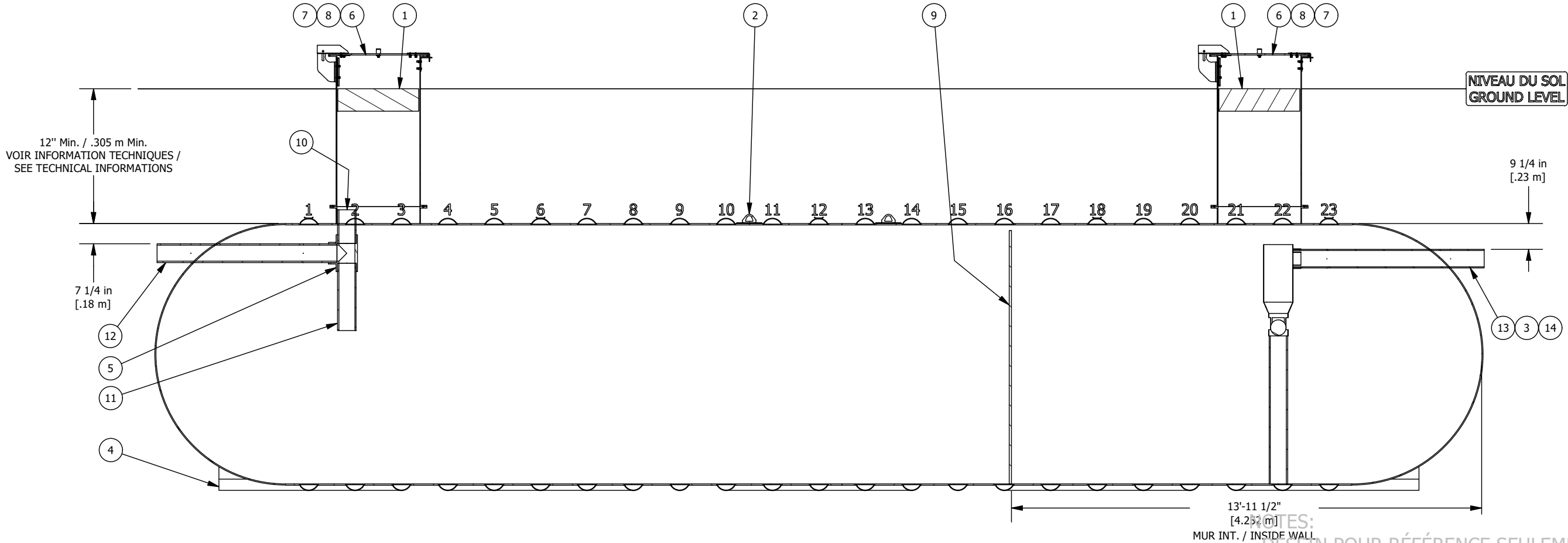
VUE D'ÉLEVATION COUPÉE CUT ELEVATION VIEW
