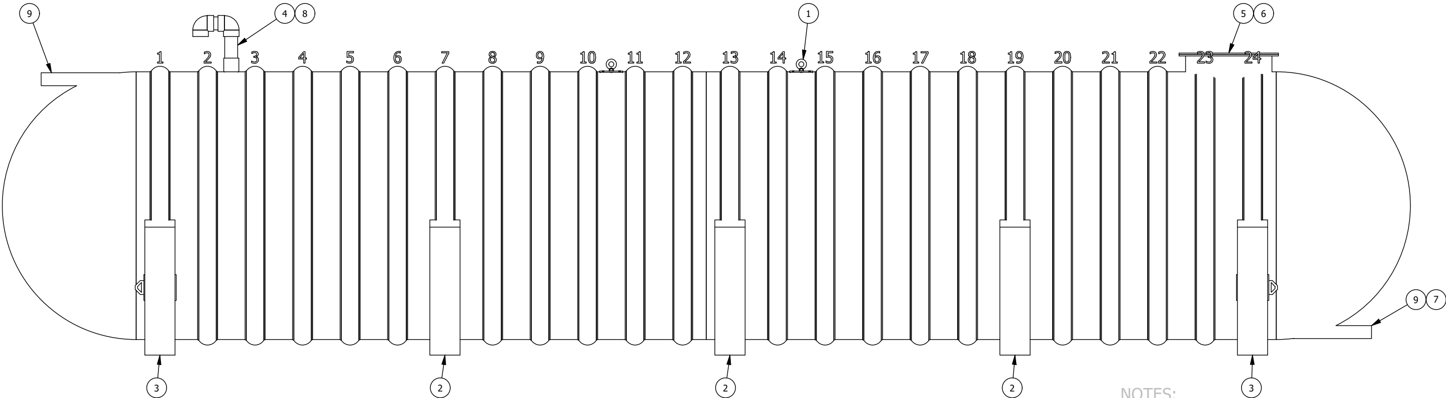
VUE D'ÉLÉVATION ELEVATION VIEW
