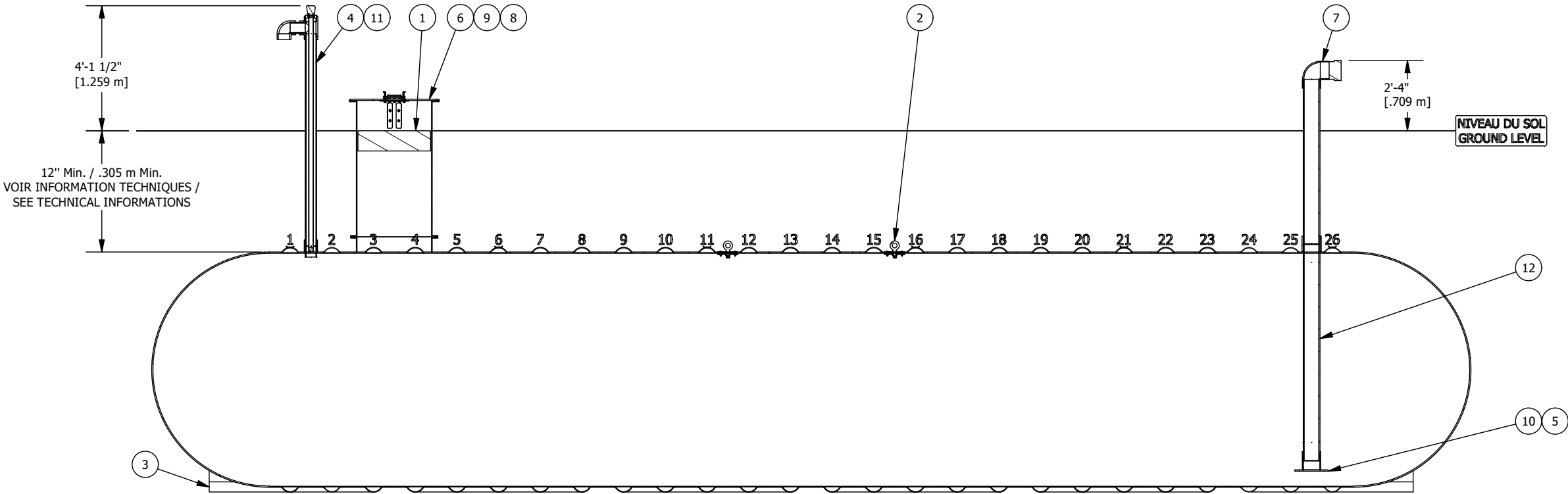
VUE D'ÉLEVATION COUPÉE CUT ELEVATION VIEW
