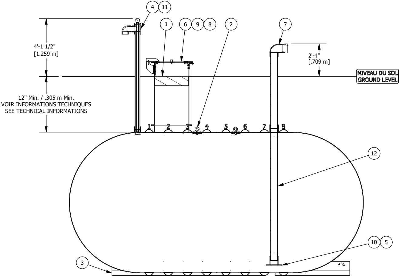
VUE D'ÉLEVATION COUPÉE CUT ELEVATION VIEW
