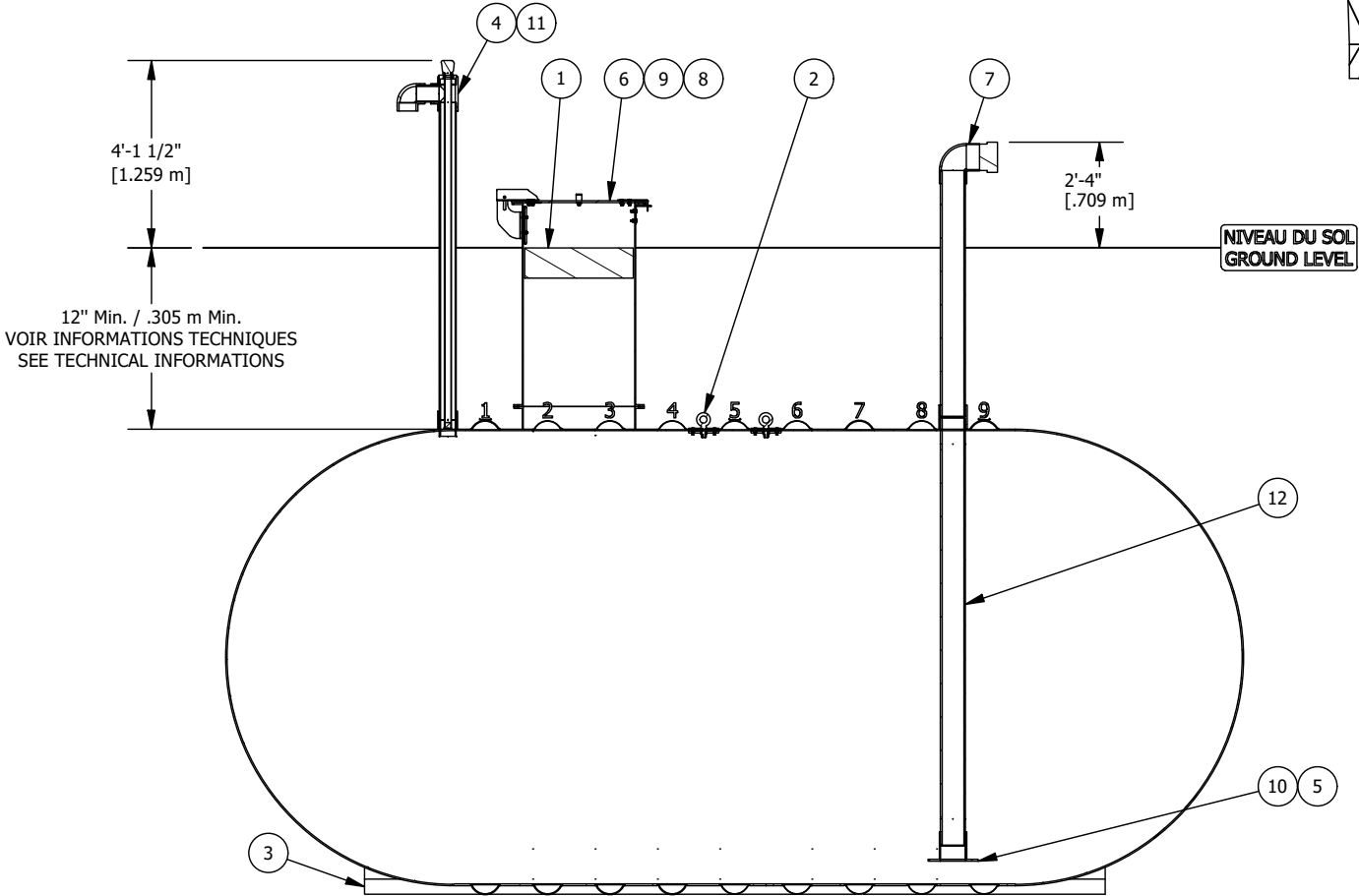
VUE D'ÉLEVATION COUPÉE CUT ELEVATION VIEW
