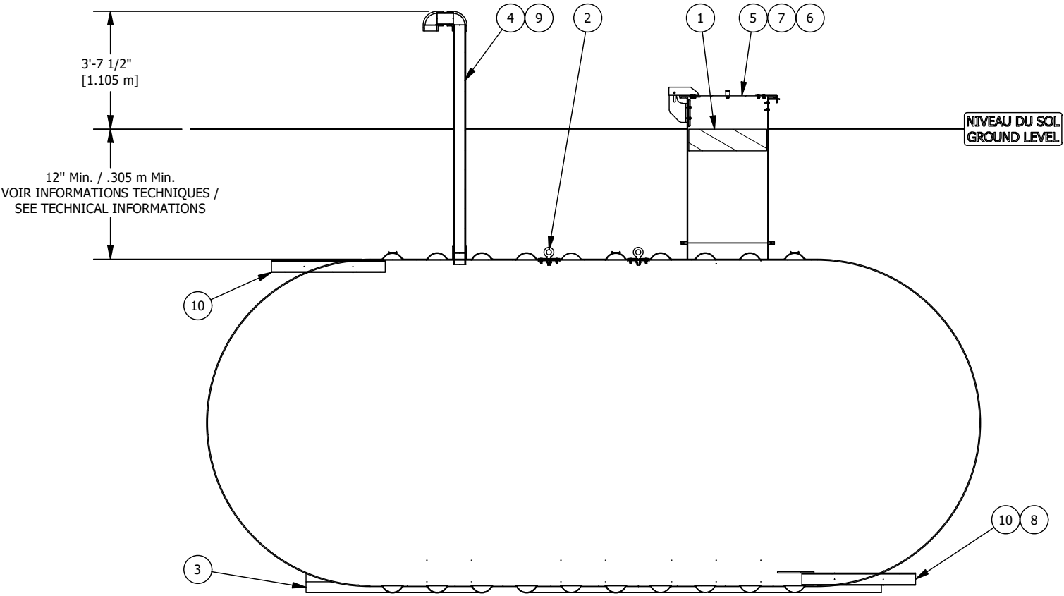
VUE D'ÉLEVATION COUPÉE CUT ELEVATION VIEW
