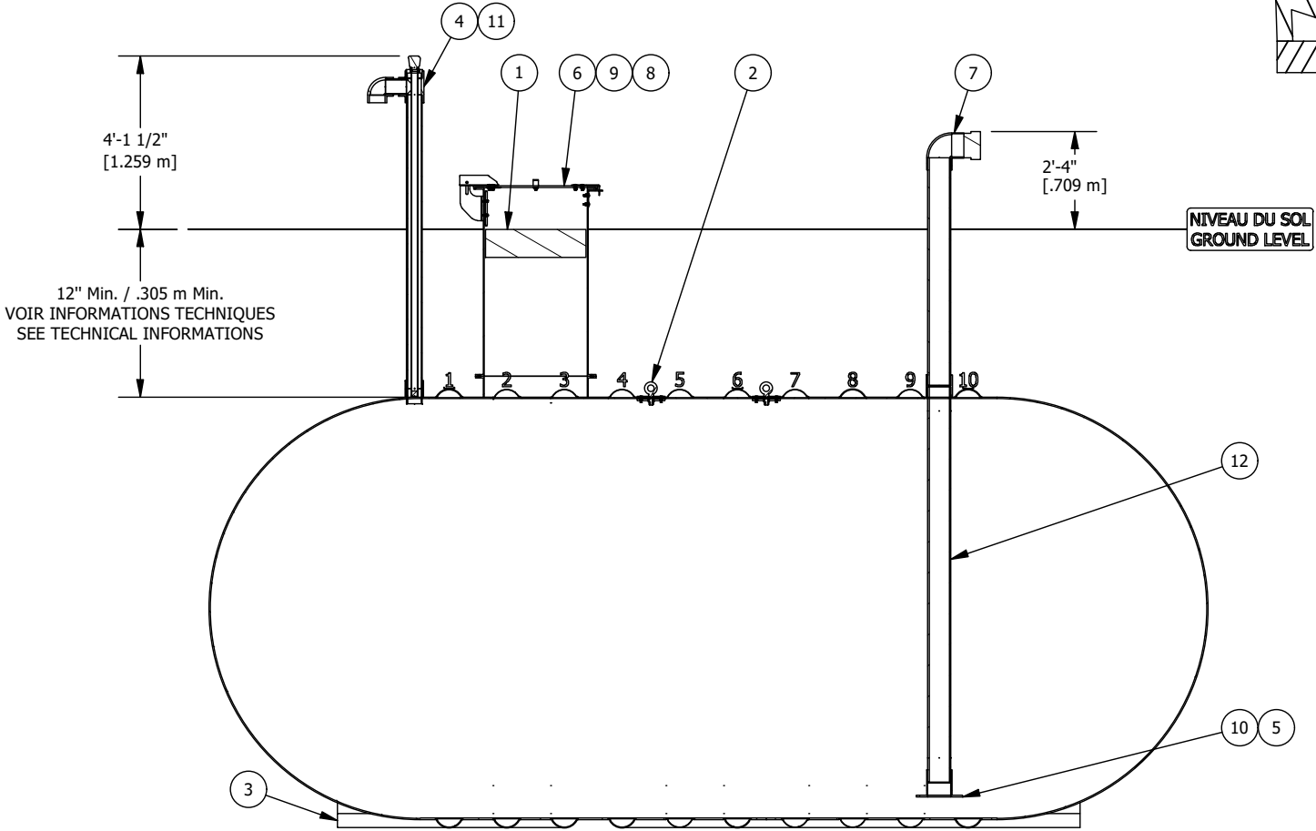
VUE D'ÉLÉVATION COUPÉE CUT ELEVATION VIEW
