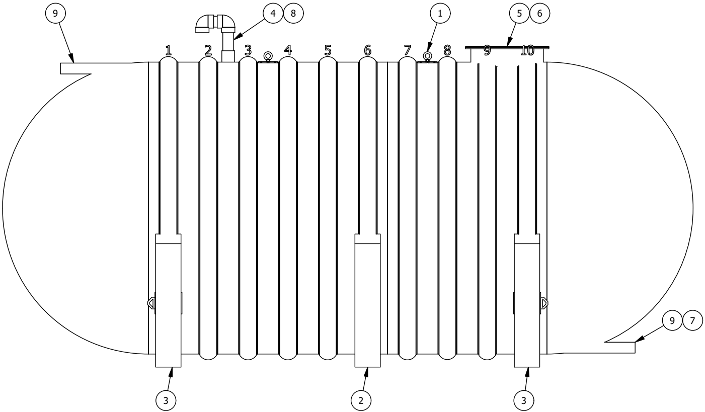
VUE D'ÉLÉVATION ELEVATION VIEW
