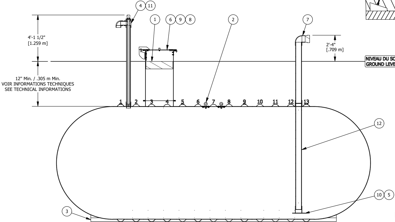
VUE D'ÉLÉVATION COUPÉE CUT ELEVATION VIEW
